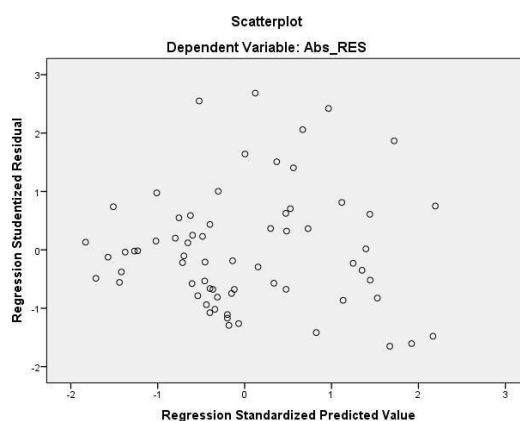
Gambar 1 Analisa grafik scatterplot
