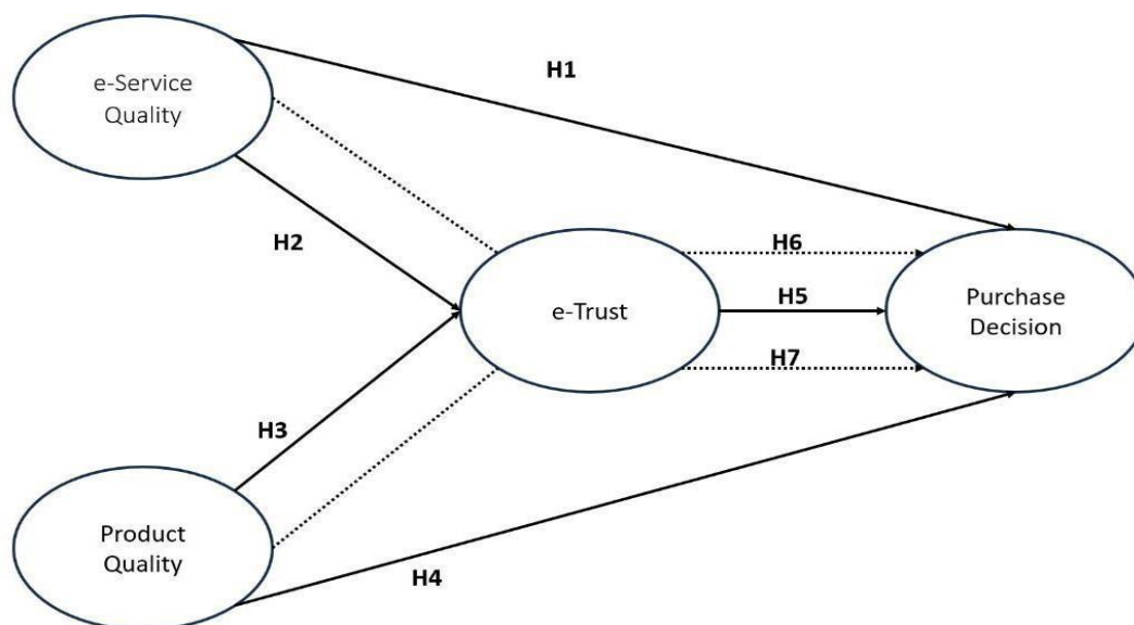
Gambar 1. Kerangka Konseptual
